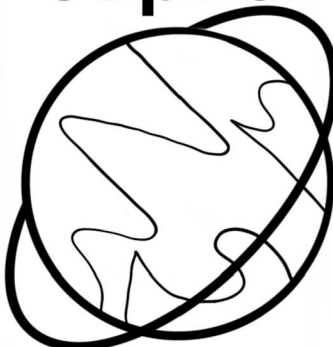
Uranus
